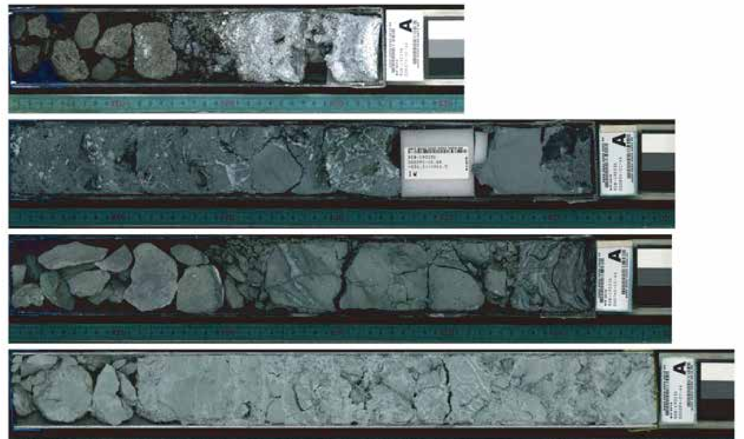
▲硫化鉱物濃集層、変質粘土層、変質火山岩層および珪化した白色粘土層の代表的なコア試料。下部(4本目)の珪化した白色粘土層のコア試料は一部分のみを抜粋。
