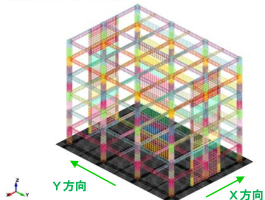
図 - 3 主架構の鉄筋解析モデル(床非表示)
