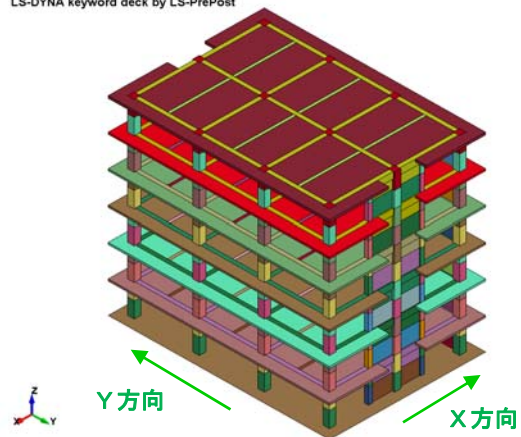
図 - 2 解析建物全体モデル(入力データのレイヤー色分け表示)
