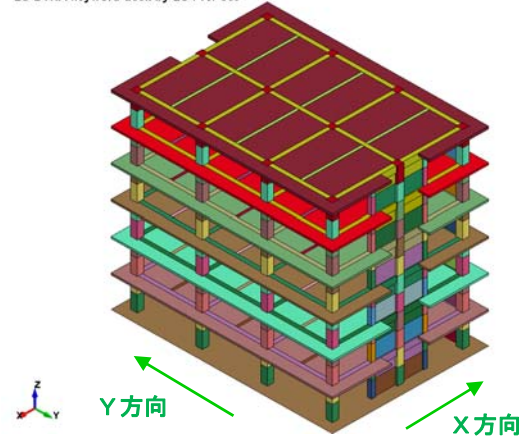
図-1 解析建物全体モデル(入力データのレイヤー色分け表示)
