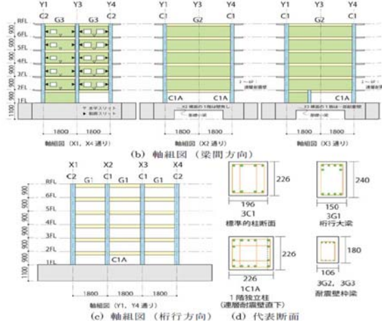
図-3 縮小6層RC造耐震壁フレーム付建物
