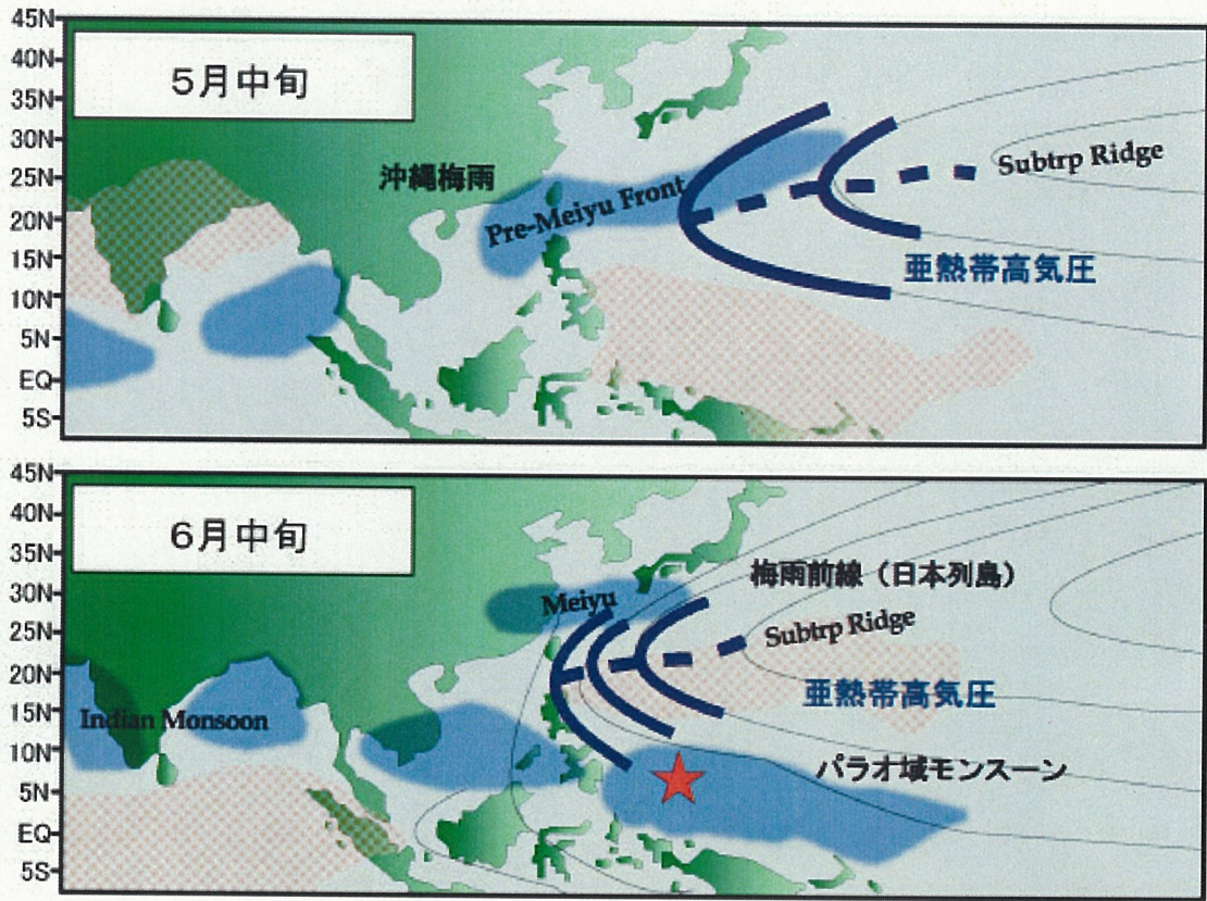
図1 日本の梅雨とパラオ域モンスーンとの関係
