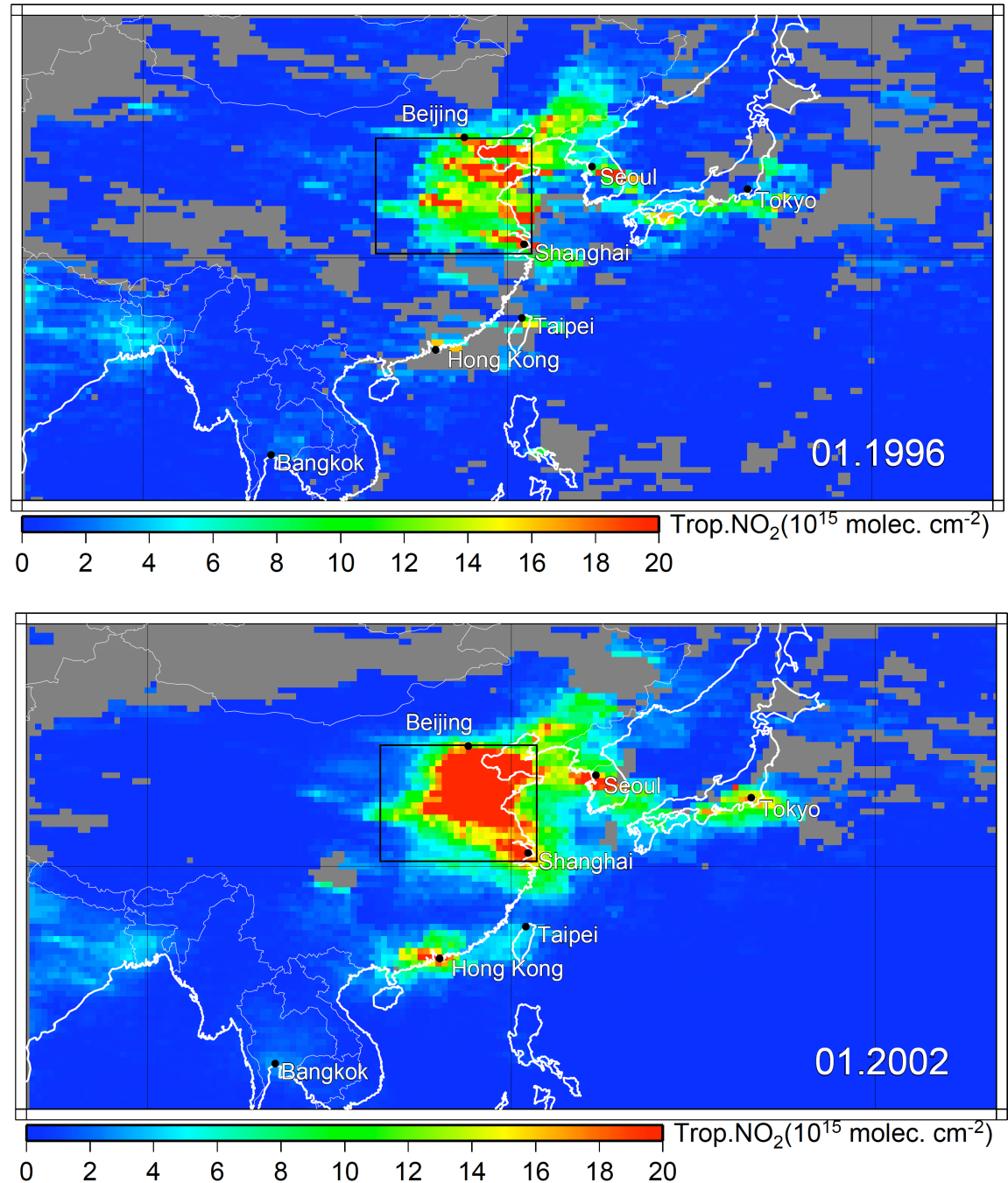
図1 : GOMEによって測定された東アジアにおけるNO 2 の対流圏濃度分布。
