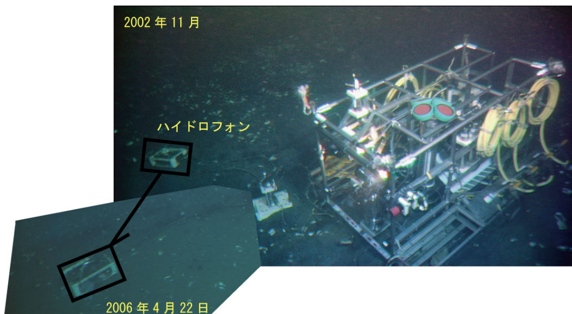
平成 18 年 4 月 21 日の地震後の泥流で、約 3m 移動したハイドロフォン
