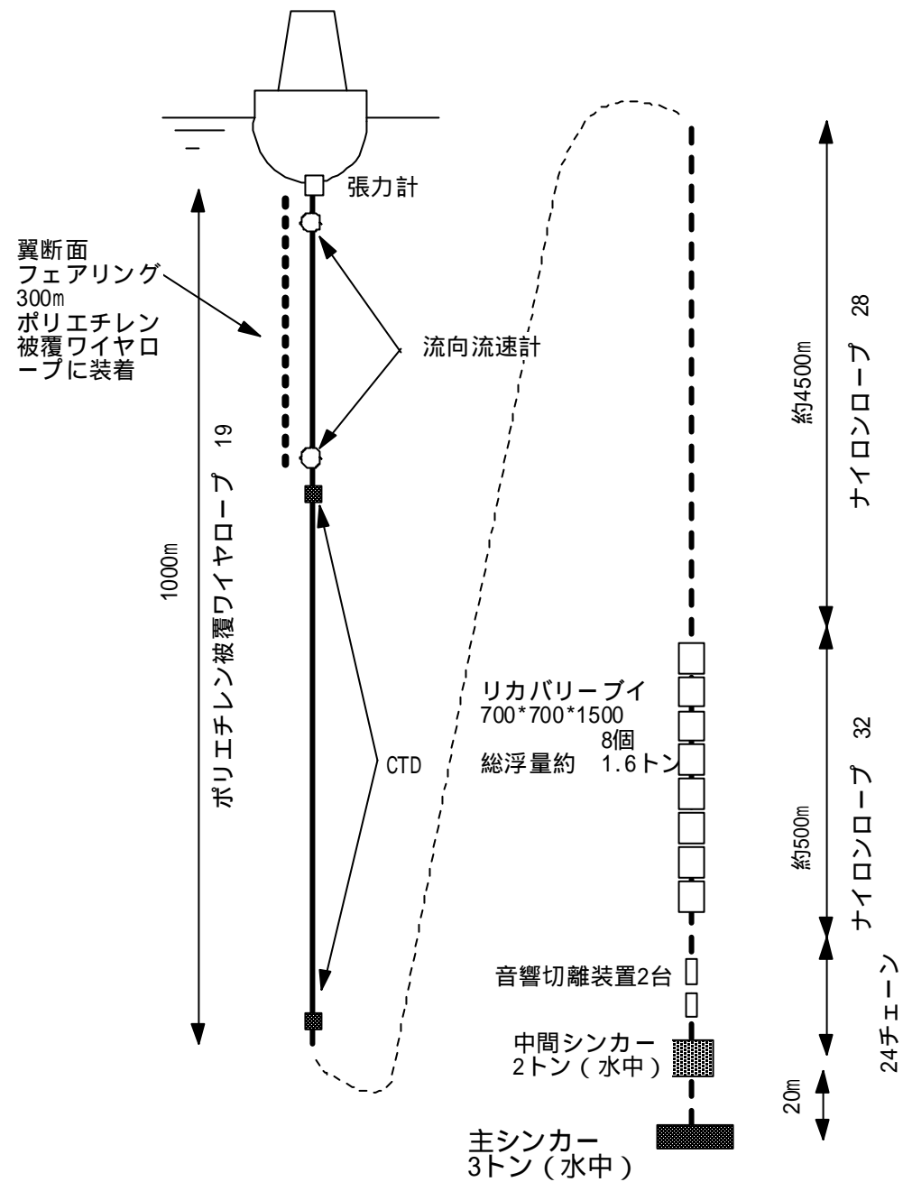
図1 中高緯度用実証機概念図
