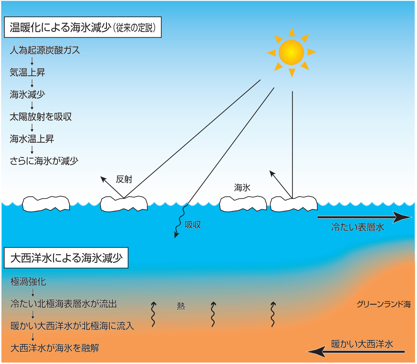
図1 海水減少のメカニズム
