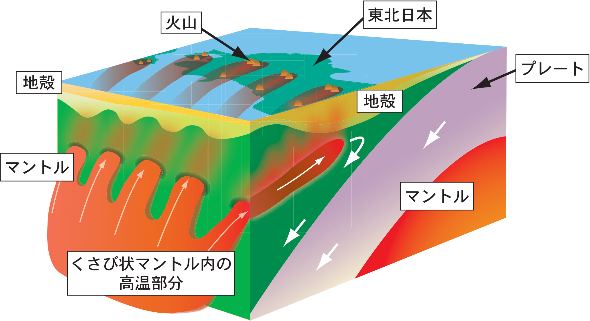
図1 マントル内の指状の高温領域と火山帯の分布
