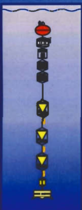
生物地球化学研究用係留系
