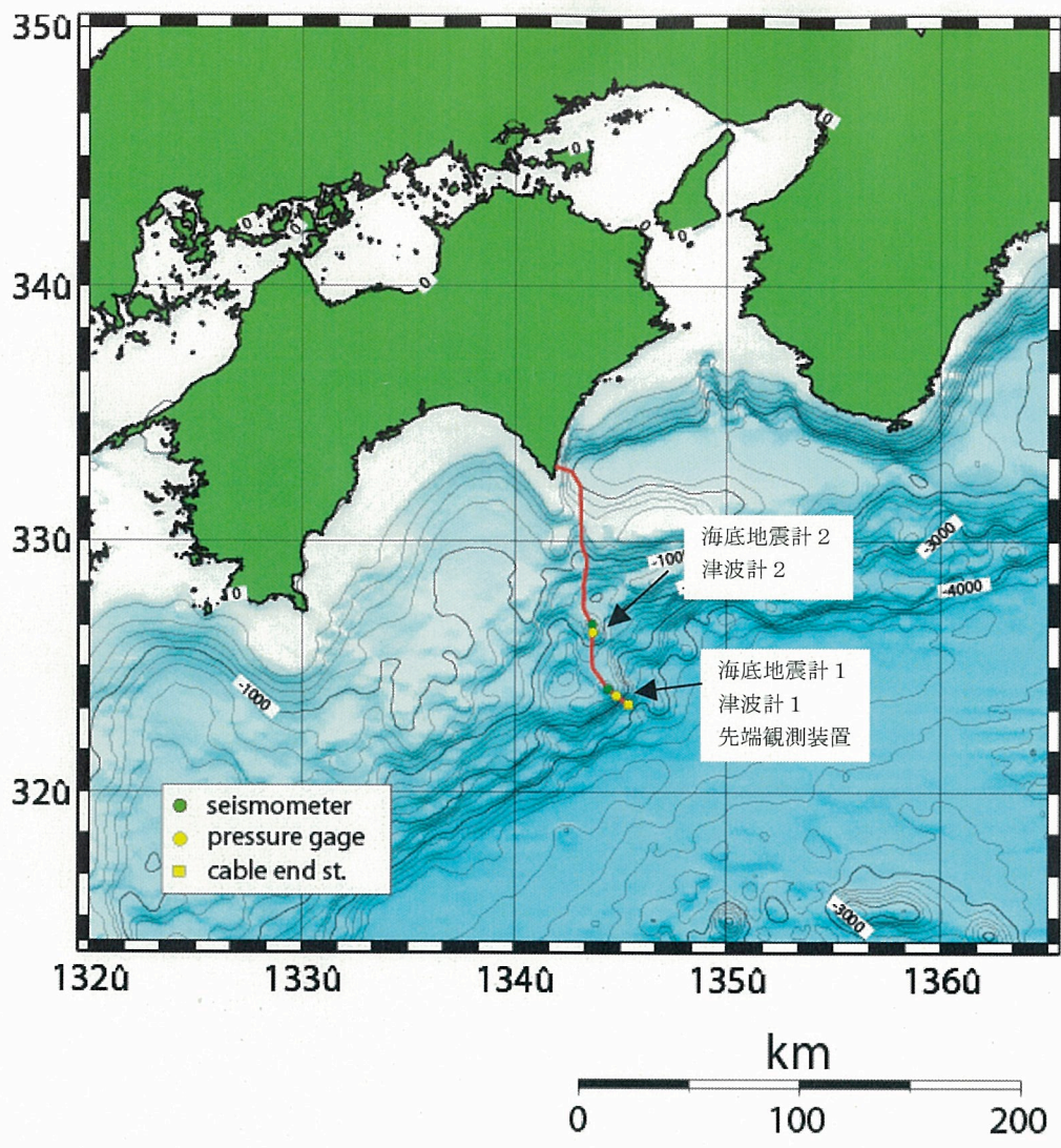
図1 高知県室戸岬沖「海底地震総合観測システム」ケーブルルートと機器の設置位置
