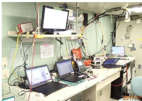
写真-6 船上局展開風景(「みらい」生物化学処理室)
