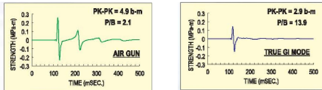
図-3 エアガン波形比較
