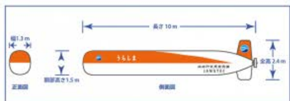
寸法
